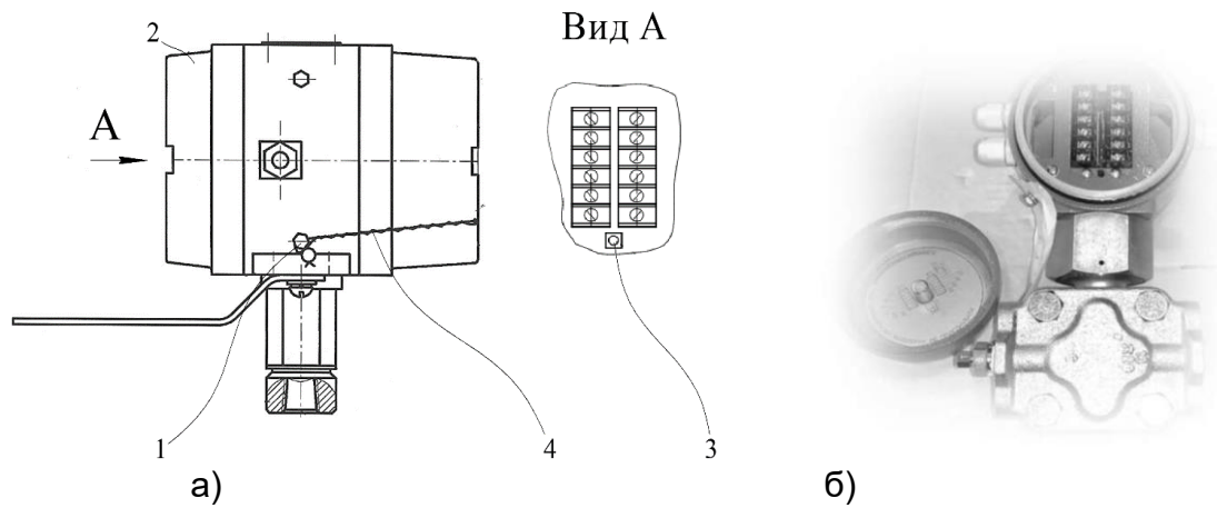
Рисунок 4. Схема пломбування Обчислювачів модифікації «ПК-В»
