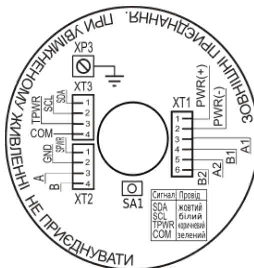
Рисунок 4.5 – Вид вигляду схем зовнішніх приєднань ПК-В з зовнішнім живленням для підключення перетворювача температури ПТ-1-Д-04 з інтерфейсом i^2C та лічильника: а) лічильник з імпульсним інтерфейсом; б) лічильник-витратомір з інтерфейсом RS485.
