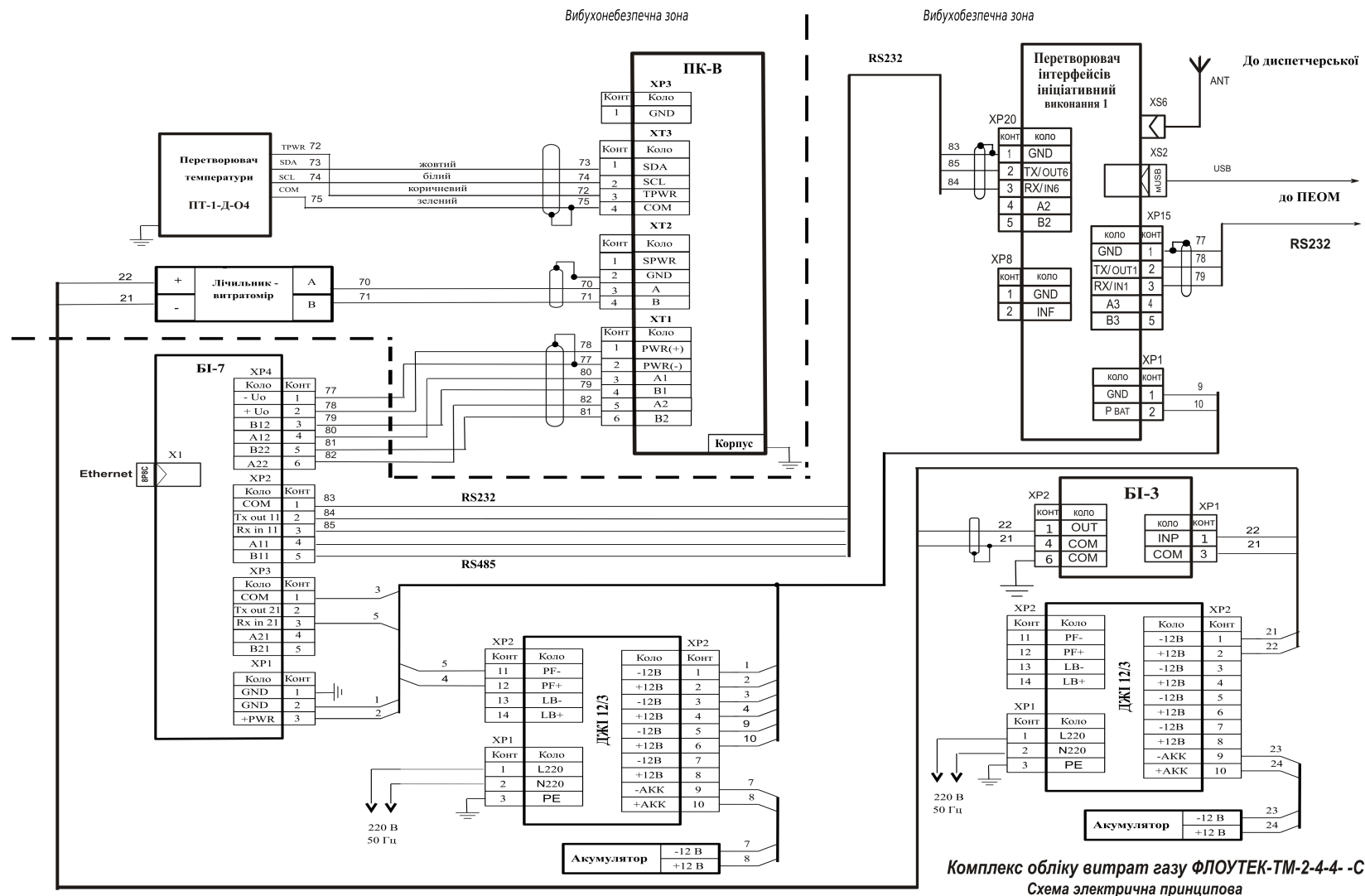
Рисунок Б.6-б – Схема підключення обчислювача ПК-В Комплексу ТМ-2-4-4- -С з цифровим лічильником-витратоміром газу та перетворювачем температури ПТ-1-Д-О4 з інтерфейсом і 2 С
