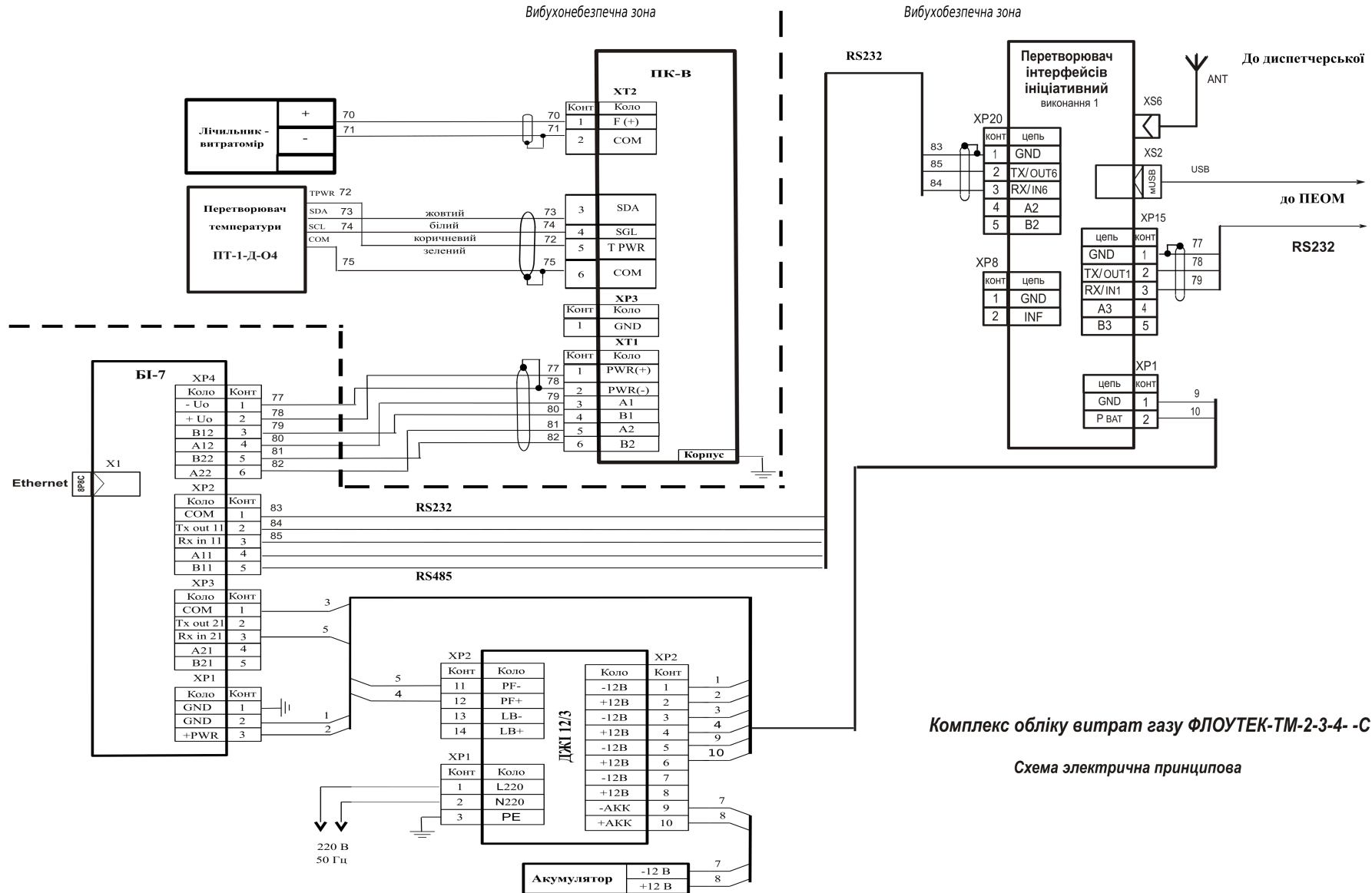
Рисунок Б.6-а – Схема підключення обчислювача ПК-В Комплексу ТМ-2-3-4- -С з імпульсним лічильником газу та перетворювачем температури ПТ-1-Д-О4 з інтерфейсом t^2C
