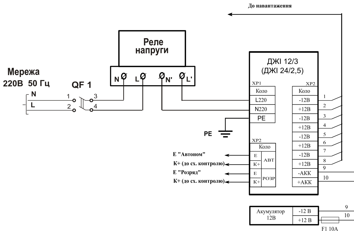
Рис 4.4. Загальна схема підключення реле напруги до ДЖІ.
