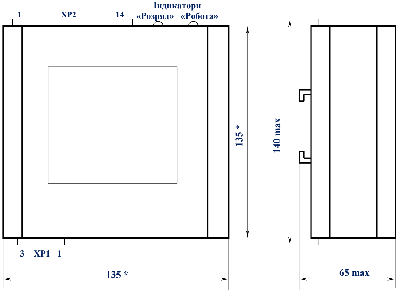
Рис. А.2. Габаритні розміри ДЖІ
