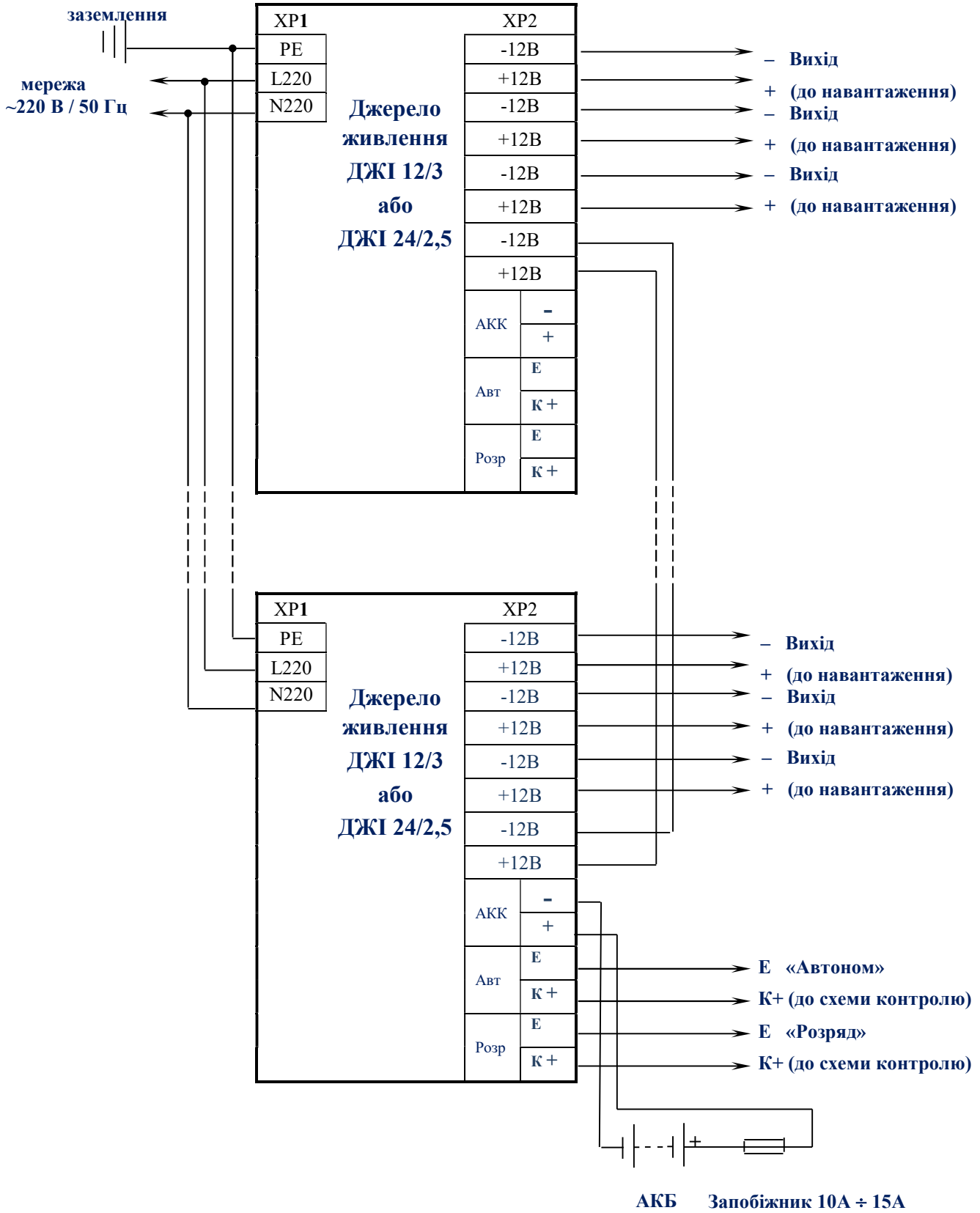
Рис. 4.2. Паралельне включення ДЖІ
