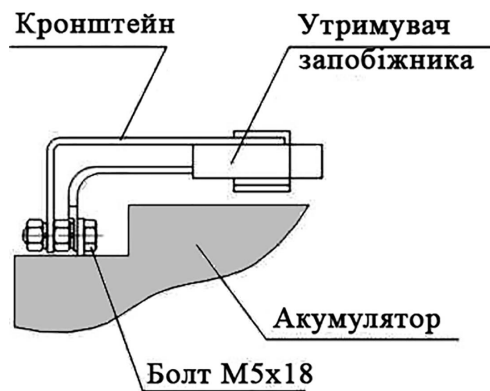
Рис. А.3. Схема кріплення утримувача запобіжника до акумулятора
